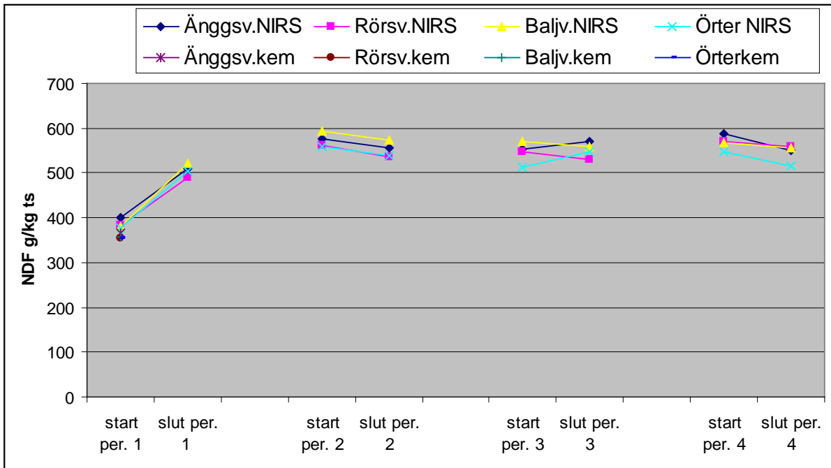
Figur 11a. Halt NDF i klippta prover 2011. Varje punkt är ett medeltal från nio provrutor. De nedre punkterna vid första provtillfället är enligt den kemiska analysen.
