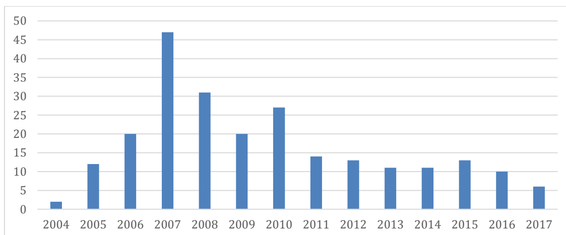
Figur 2. Antal nya besättningar med fall av fotröta per år för åren 2004-2017
